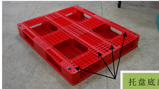
(托盘反面图)
