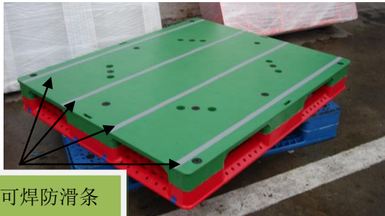
(托盘正面图)
